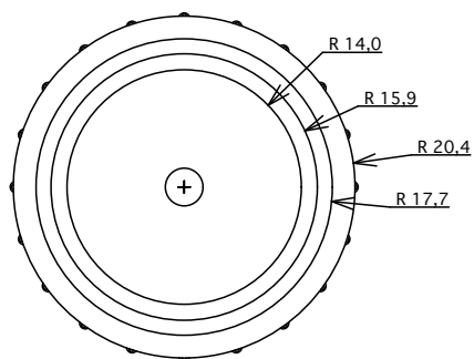
felülnézet
