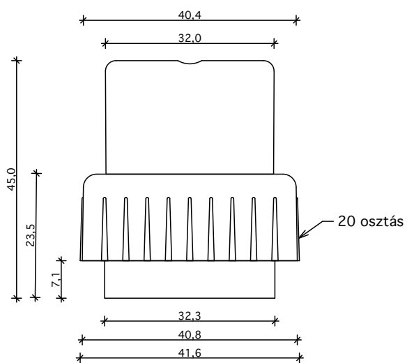
oldalnézet
