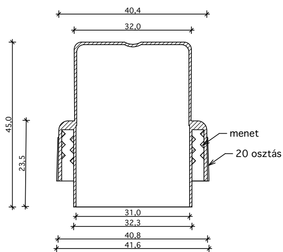
metszet
