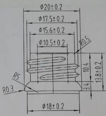
口部详细 2:1
