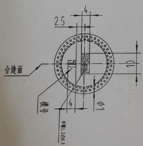
B向视图
