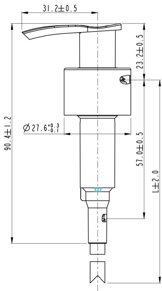
Section A-A Scale 1.000
