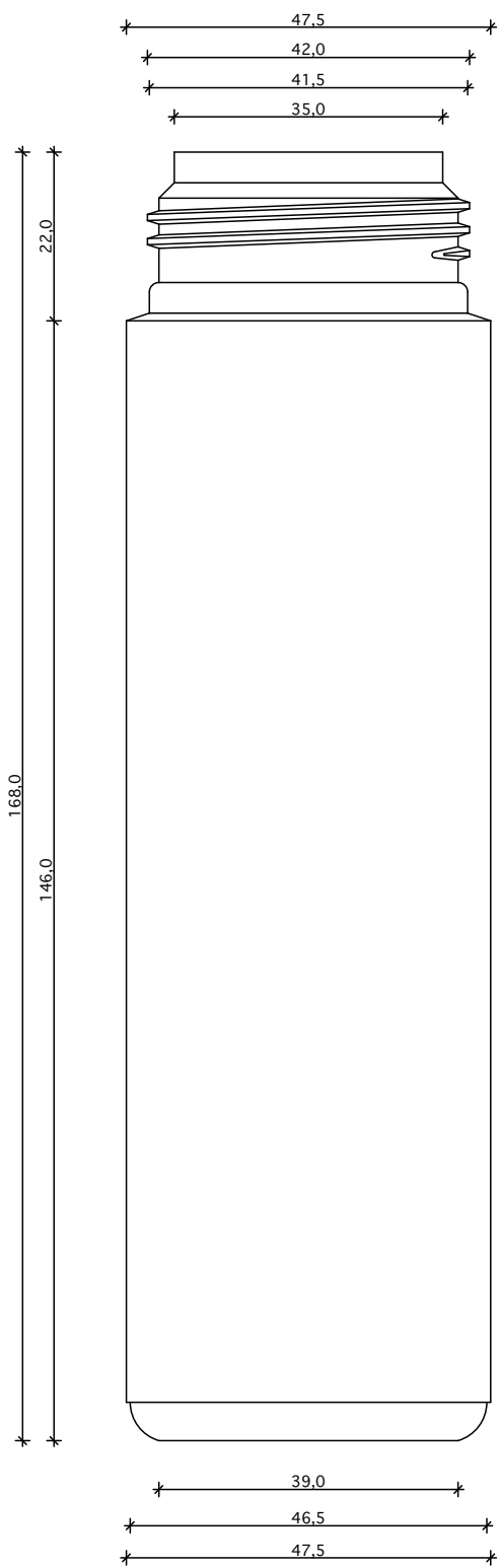
oldalnézet
