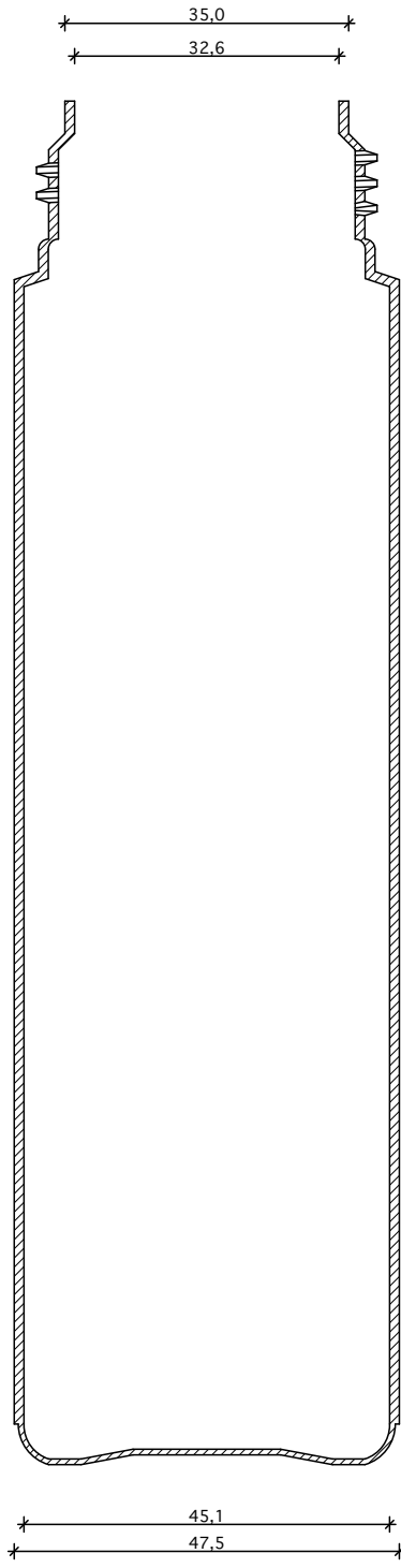
metszet
