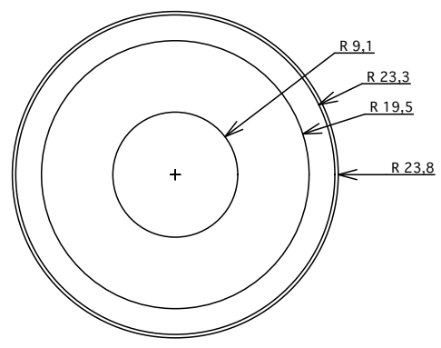
alulnézet
